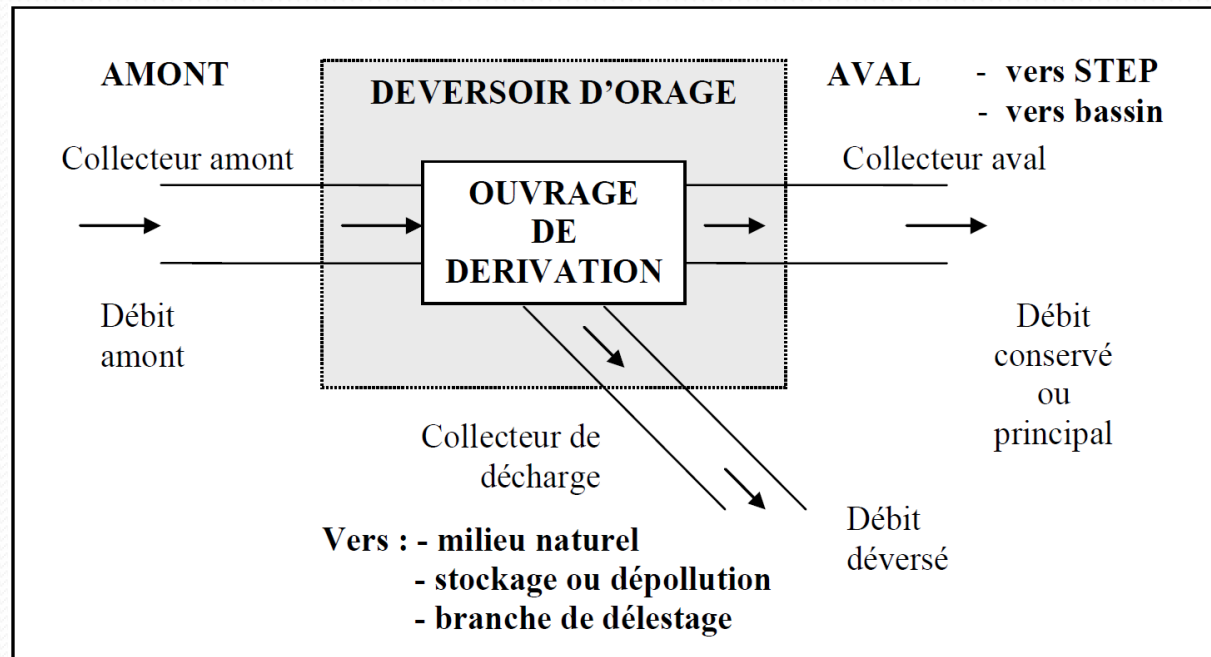
Schéma de principe du déversoir d'orage
