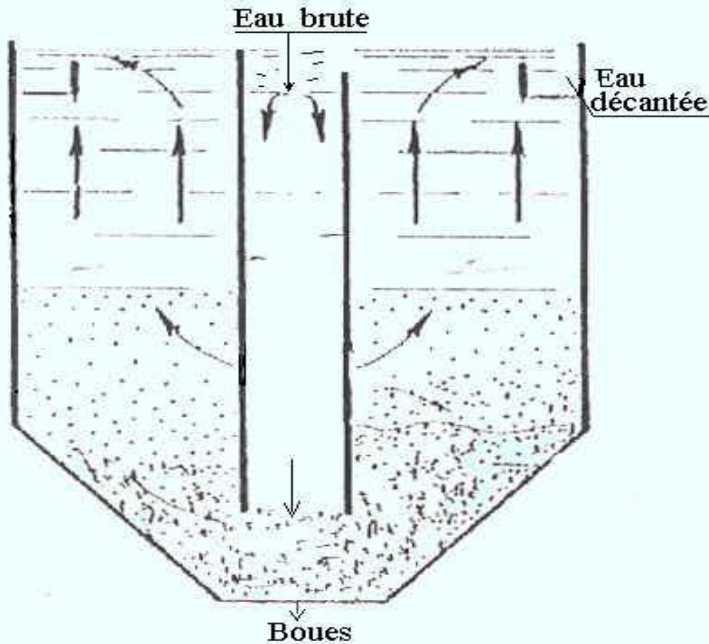
décanteur statique
