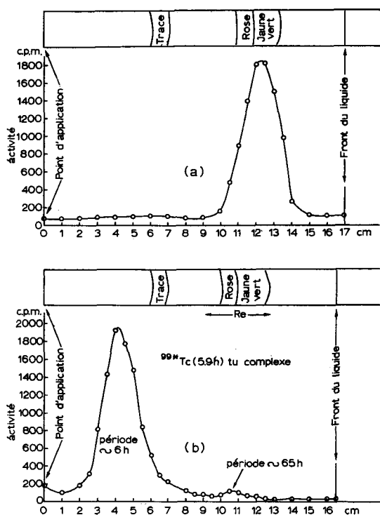
Fig. 12. Distribution de l'activité et des taches révélées avec \text{SnCl}_2 -KCNS: (a) d'une solution de ^{99m}\text{TcO}_4^- (avec du Mo comme impureté) et (b) la même solution après addition de quelques mg de thiourée. L'endroit où se trouve le Re est indiqué sur la figure.
