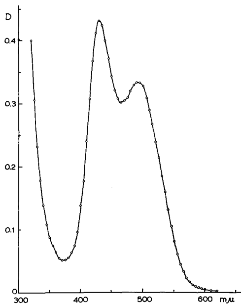
Fig. 10. Spectre d'absorption d'un mélange TcO_4^- - ReO_4^- dans HNO_3 2 N avec une addition d'un excès de thiourée. Le spectre a été mesuré après une dilution avec 0.5 N HCl contenant 1 % de thiourée.
