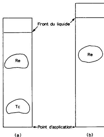
Fig. 11. (a) Un chromatogramme d'une mélange \text{TcO}_4^- - \text{ReO}_4^- en \text{HNO}_3 2 N avec un excès de thiourée, développé avec HCl 2 N . (b) Un chromatogramme de \text{ReO}_4^- seul mélangé avec la thiourée dans \text{HNO}_3 2 N et laissé au repos pendant 16 heures.
