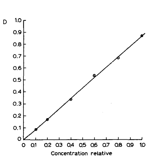
Fig. 6. Graphique de la densité optique contre la concentration (relative) (vérification de la loi de Beer). Substance: complexe jaune Re-thiourée. Longueur d'onde 390 m \mu , ouverture de 0.036 mm, cellule de verre d'une épaisseur de 1 cm.
