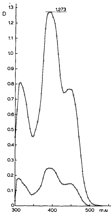
Fig. 5. Le spectre d'absorption du complexe jaune du rhénium avec la thiourée dans \text{HCl} 0.5 N contenant 1 % de thiourée dans deux dilutions différents.
