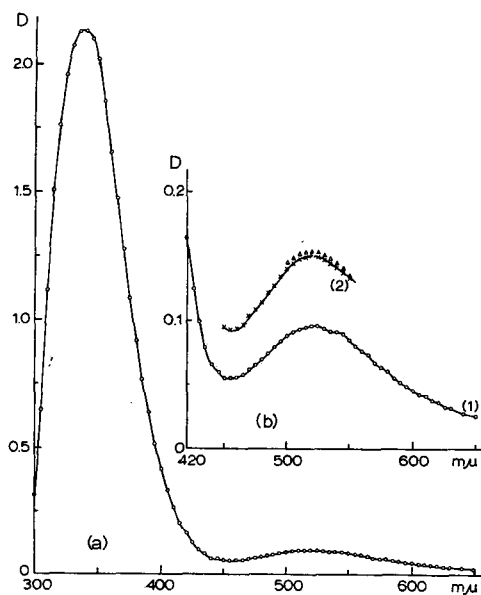
Fig. 4. Le spectre d'absorption du complexe pourpre rhénium-thiourée formé à partir de 0.97 mg de Re avec 4 mg de thiourée et une addition de 0.004 ml de \text{SnCl}_2 M/2 . La solution a été diluée à 3.5 ml avec \text{HCl} 0.5 N contenant 1 % de thiourée. Fig. 4b (1) est le pic du spectre de Fig. 4a à une plus grande échelle. Fig. 4b (2) la solution avec une addition de 0.006 ml de \text{SnCl}_2 M/2 . Spectrophotomètre: Unicam SP 500 avec les cellules en verre de 1 cm épaisseur.
