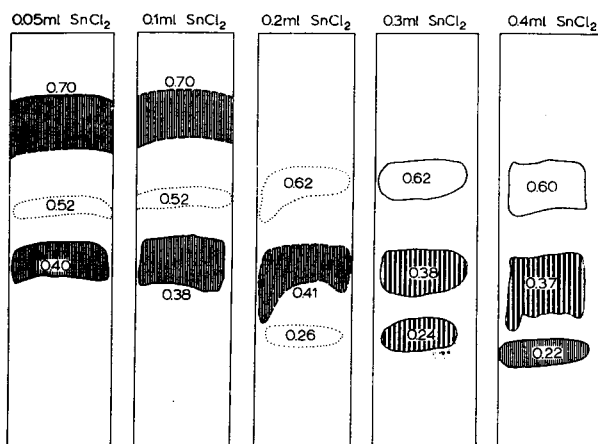
Fig. 2. Les chromatogrammes des mélanges d'une solution perrhéate-thiourée comme dans Fig. 1 avec 0,5, 1, 2, 3 et 4 équivalents de \text{SnCl}_2 (dans \text{HCl} 2 N ).
