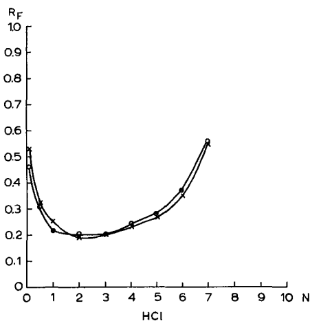
Fig. 8. Valeurs de R_F du complexe jaune de Re-thiourée et du complexe Tc-thiourée sur papier Whatman No. 1 avec comme solvant HCl aqueux. \times-\times Re; \circ-\circ Tc.
