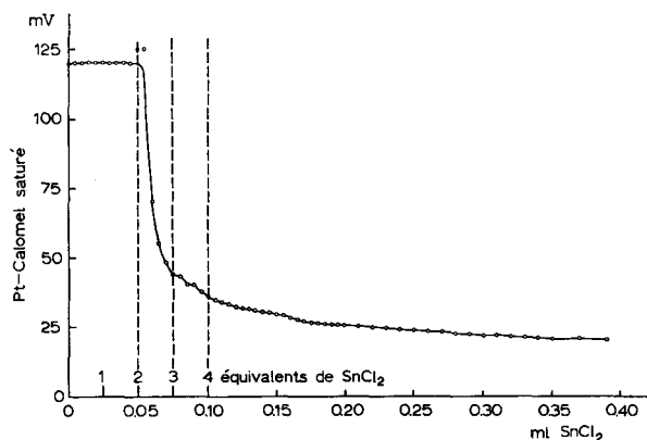
Fig. 1. Titrage de 0,1 mmole de perrhénate-20 mg thiourée dans 2 ml de HCl 2 N avec M / z \text{SnCl}_2 (précisément M/2 \times 0,94 ) (dans HCl 2 N ). Électrode: Pt/calomel saturé.
