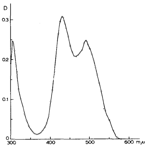
Fig. 7. Spectre d'absorption du complexe Tc-thiourée dans HCl 0.5 N contenant 1% de thiourée. Conditions comme dans Fig. 4.
