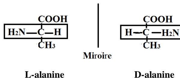
Figure 43 : structure des isomères optiques de l'alanine.
