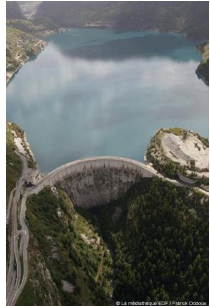
Barrage de Tignes et Lac du Chevril (Savoie)
