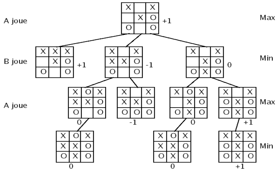
Figure 14. Arbre des niveaux de jeu de la configuration de la figure 10.
