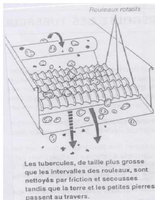
Système de nettoyage à rouleaux crenels
