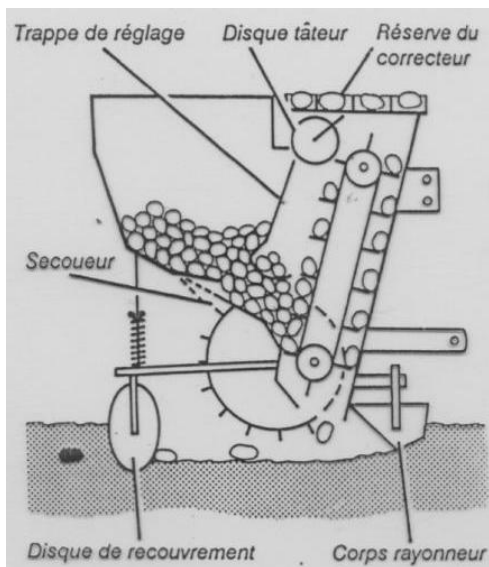
Vue en coupe d'une planteuse de pomme de terre
