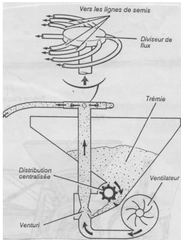
Coupe transversale d'un semoir pneumatique à distribution centralisée
