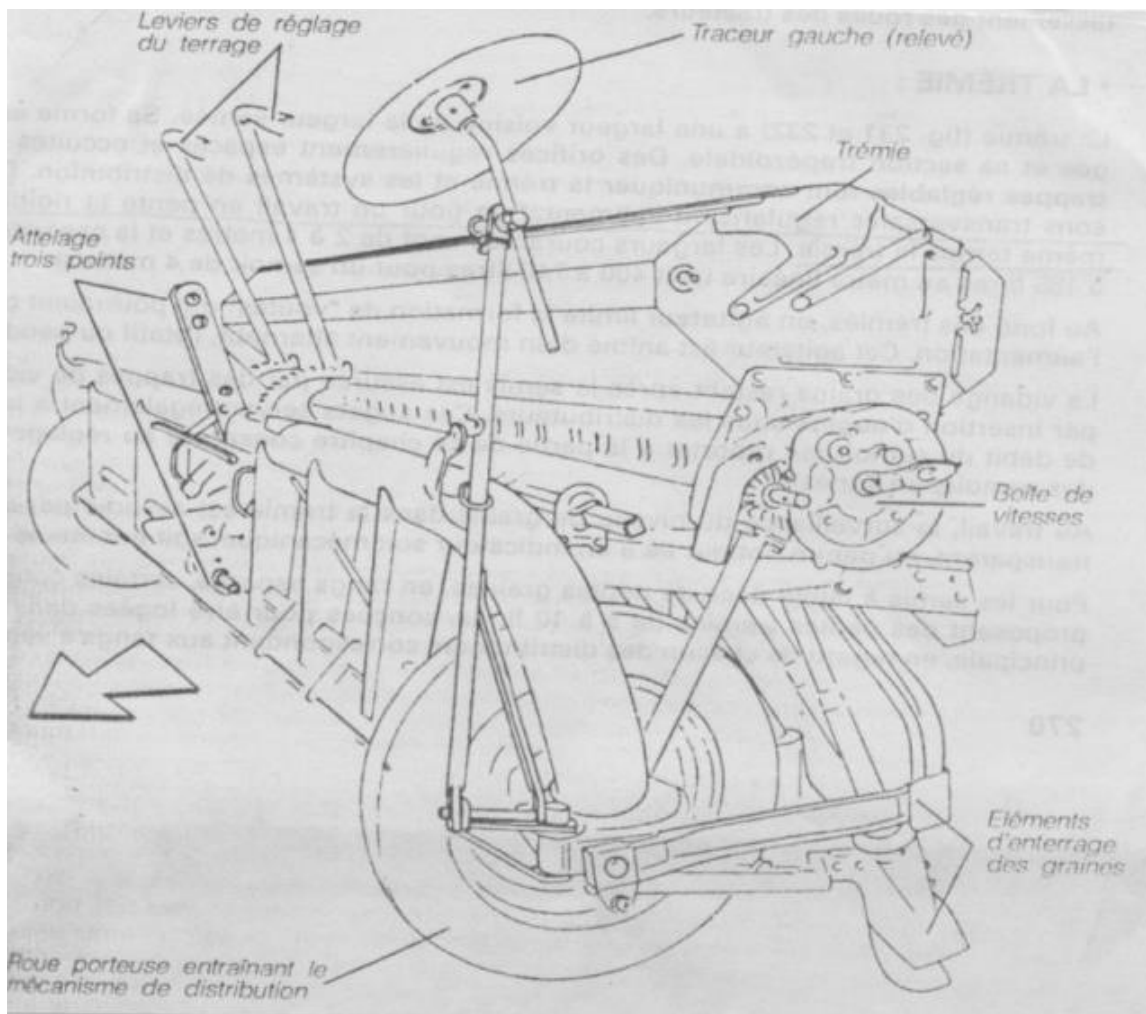
Vue générale d'un semoir en ligne à distribution mécanique
