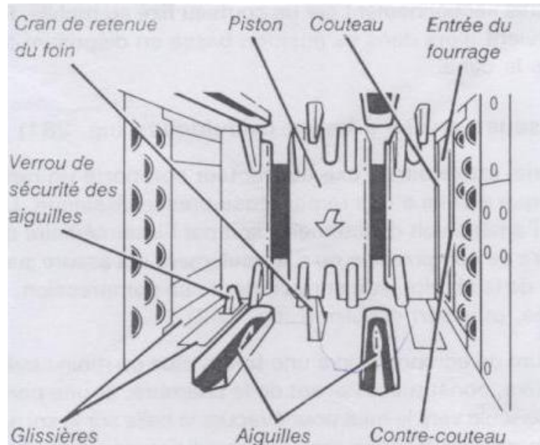
Vue intérieure du canal de compression d'une ramasseuse presse
