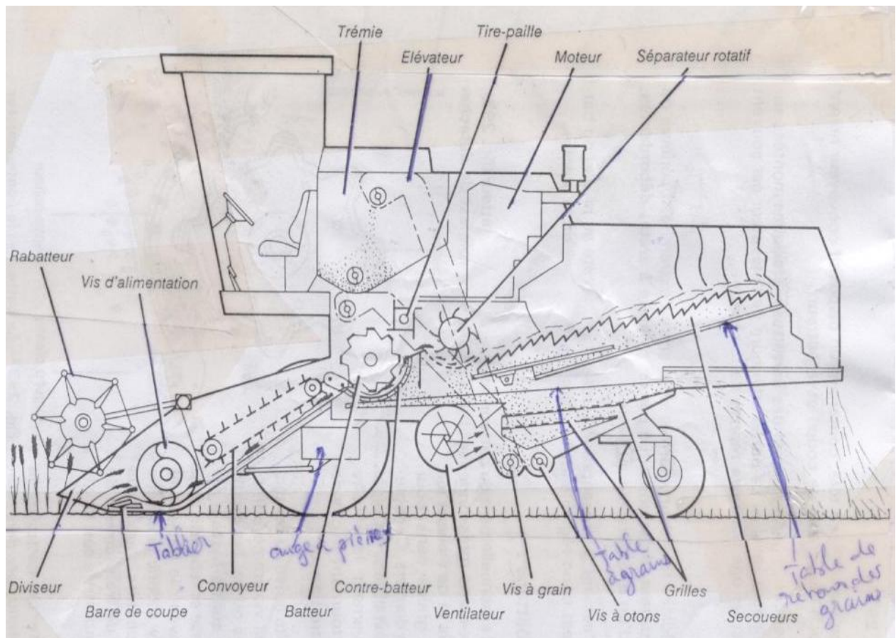
Vue en coupe d'une moissonneuse batteuse
