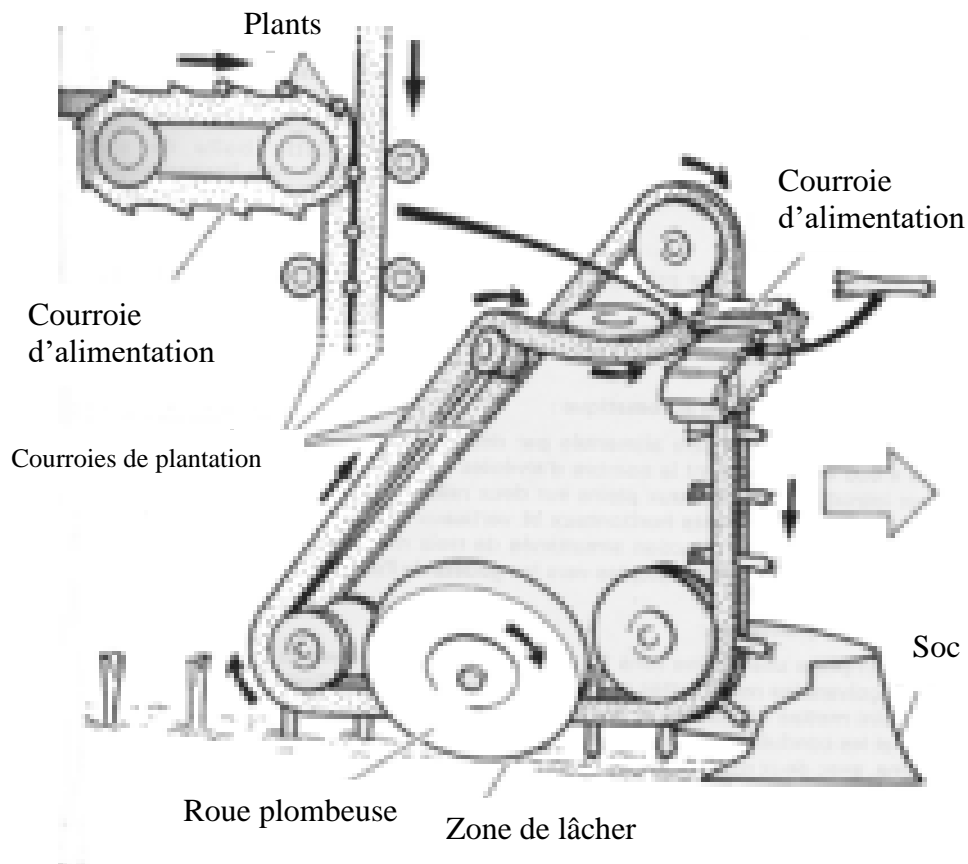
Principe d'une planteuse à courroies
