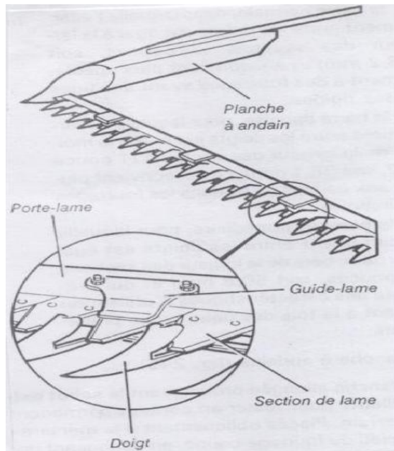
Vue générale d'une faucheuse alternative
