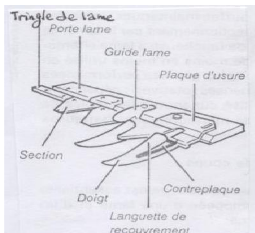
Vue partielle de la barre de coupe d'une faucheuse alternative
