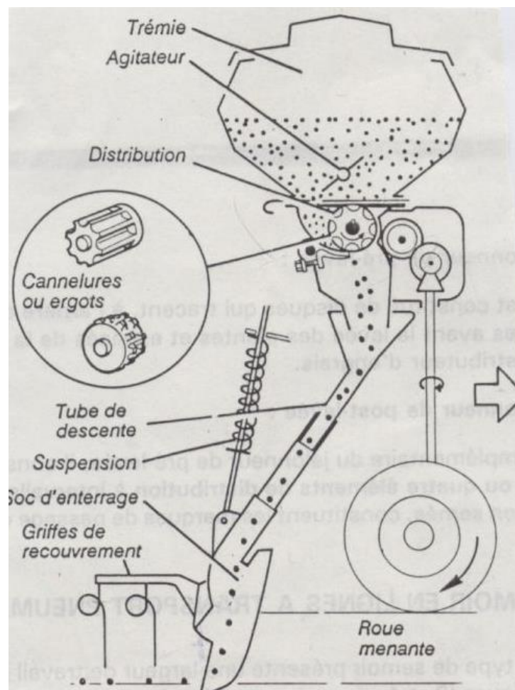
Vue en coupe et principe de fonctionnement d'un semoir en ligne à distribution mécanique.
