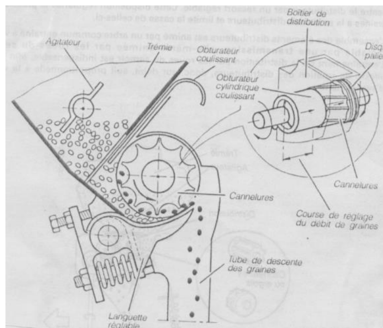
Distributeur à cannelures
