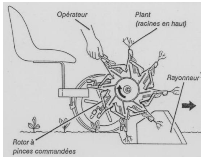
Principe d'une planteuse à roues et pinces
