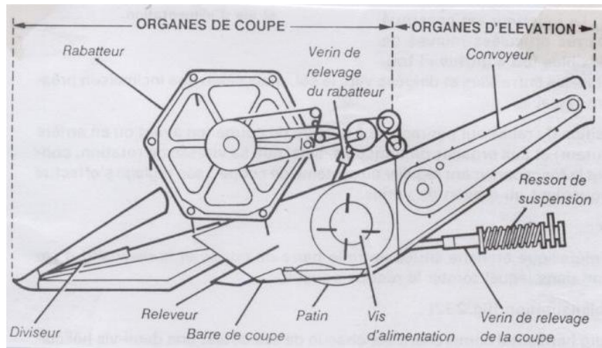
Vue des organes de coupe et d'élévation
