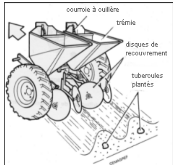
vue générale d'une planteuse de pomme de terre
