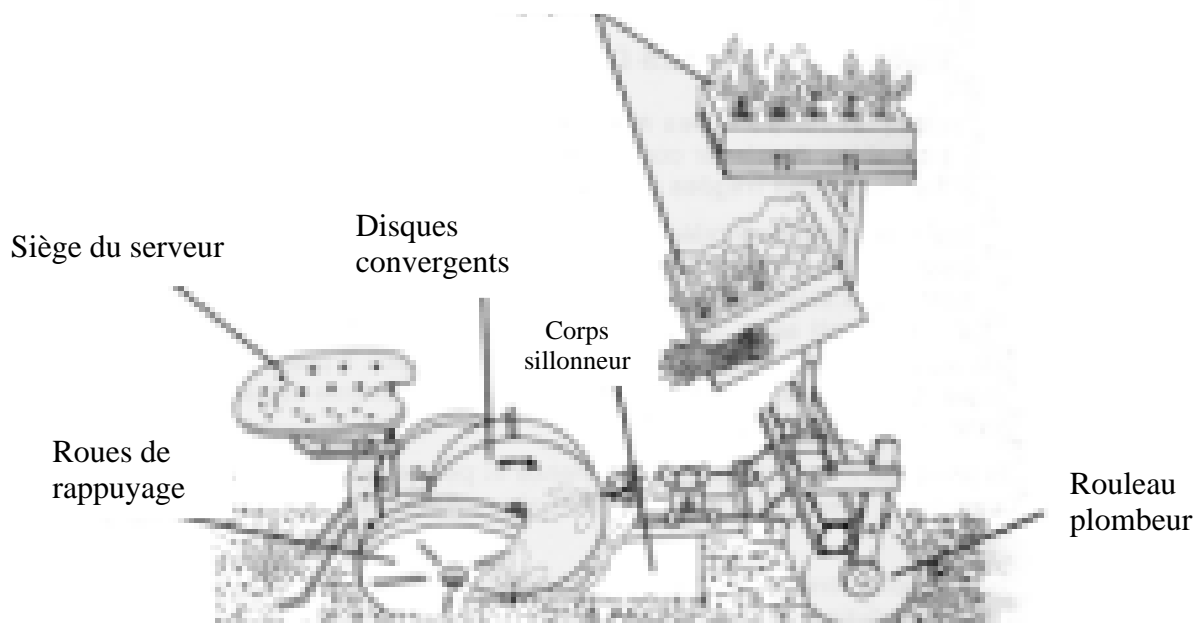
Principe d'une planteuse à disques convergents
