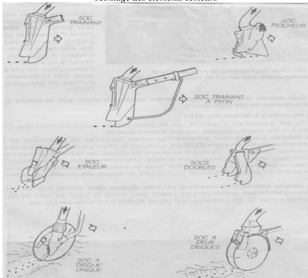
Différents types d'éléments rayonneurs
