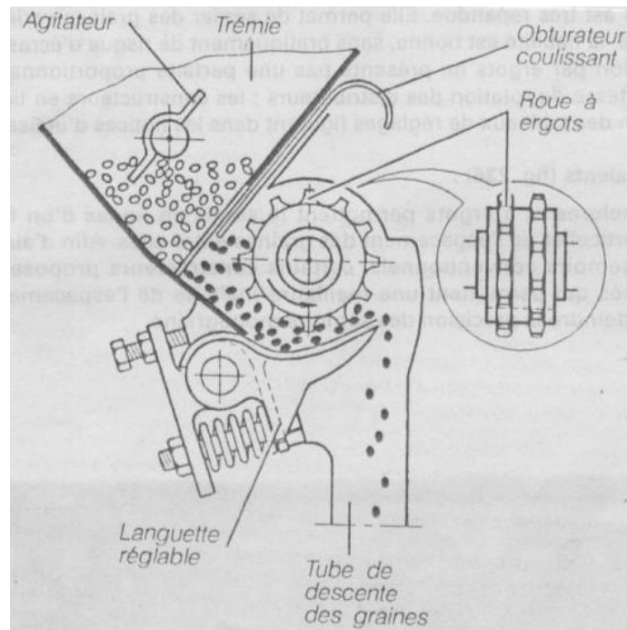
Distributeur à ergots
