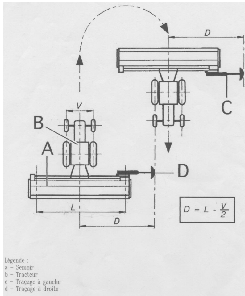
Réglage des traceurs
