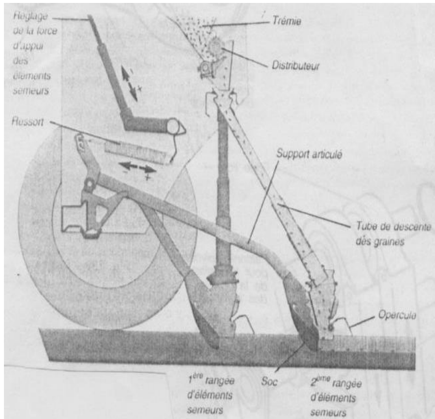
Montage des éléments semeurs
