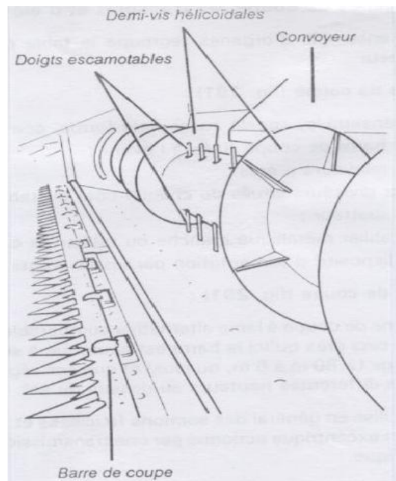
Vue de la barre de coupe et vis d'alimentation
