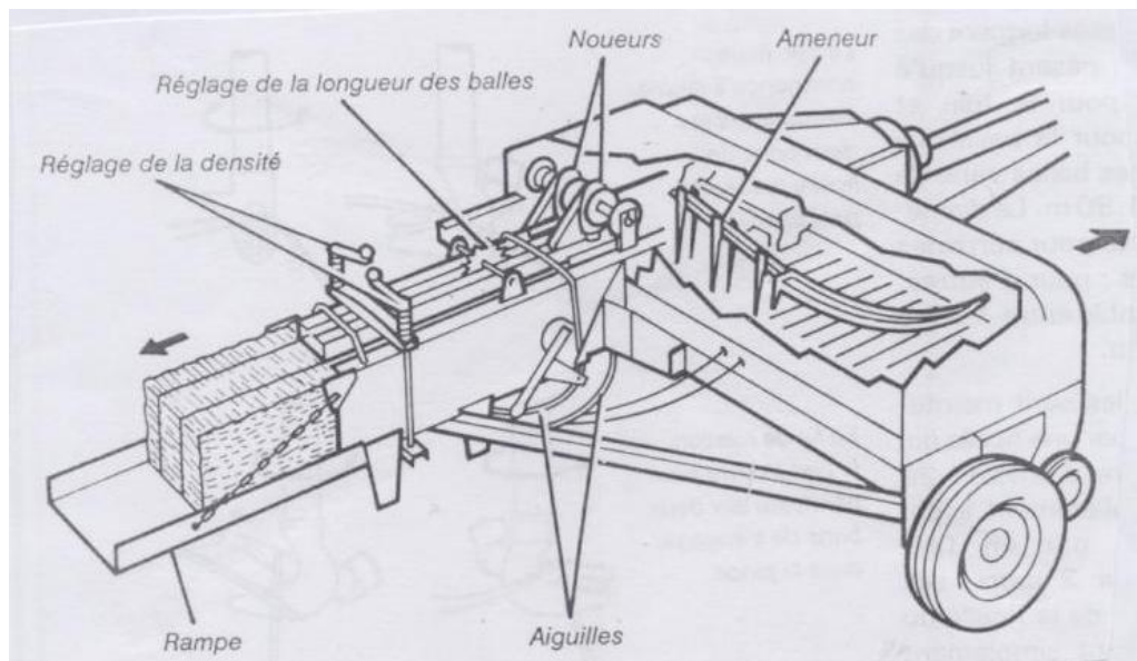
Constitution d'une ramasseuse presse à balles parallélépipédiques
