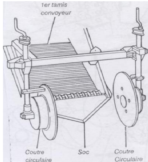
Dispositif d'arrachage et de tamisage des tubercules
