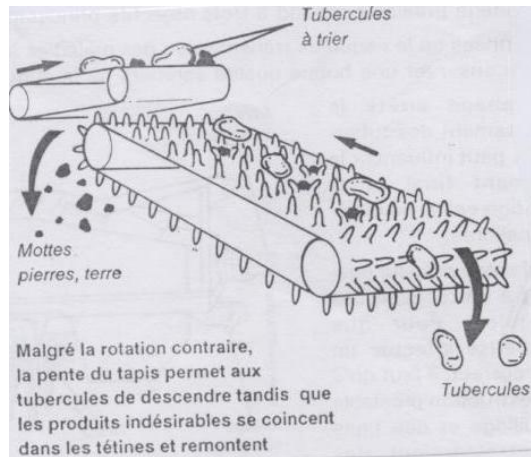
Tapis de triage à tétines en caoutchouc
