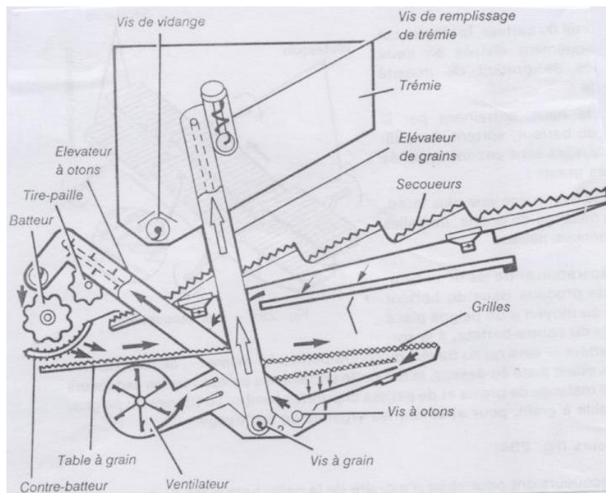
Vue des organes de battage, séparation, nettoyage et récupération des grains
