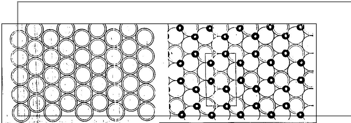
Fig 05 : Couche compacte d'hydroxyles Couche compacte d'oxygène et d'hydroxyles
