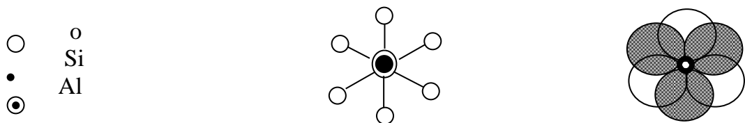
Fig. 8: Disposition Octaédrique .Elle montre la constitution d'un octaèdre. Les trois cercles supérieurs appartiennent à une couche compacte supérieur les trois autres appartiennent à une couche compacte inférieur
