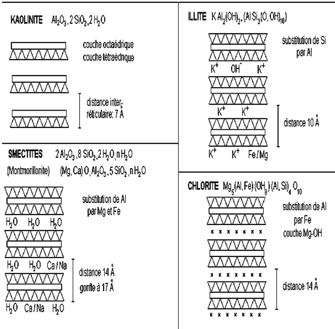
Fig :9 . représentations schématiques des structures des principaux minéraux phylliteux
