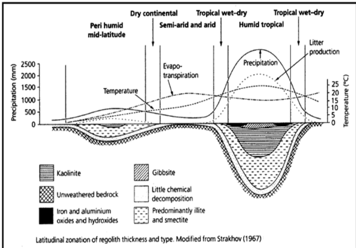
fig 12 Hydrolyse et zonation climatique (Allen, 1997).
