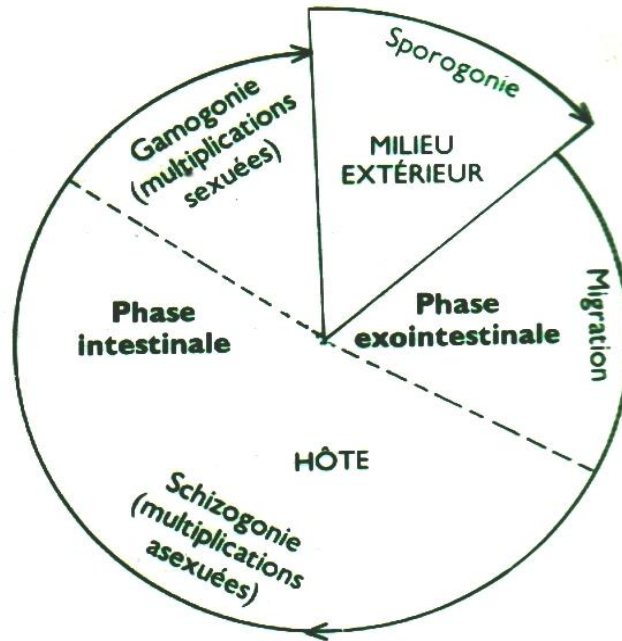
Figure 1 : Représentation schématique des étapes du cycle évolutif des coccidies (Yvoré et al., 1982). Cycle évolutif monoxène direct long.
