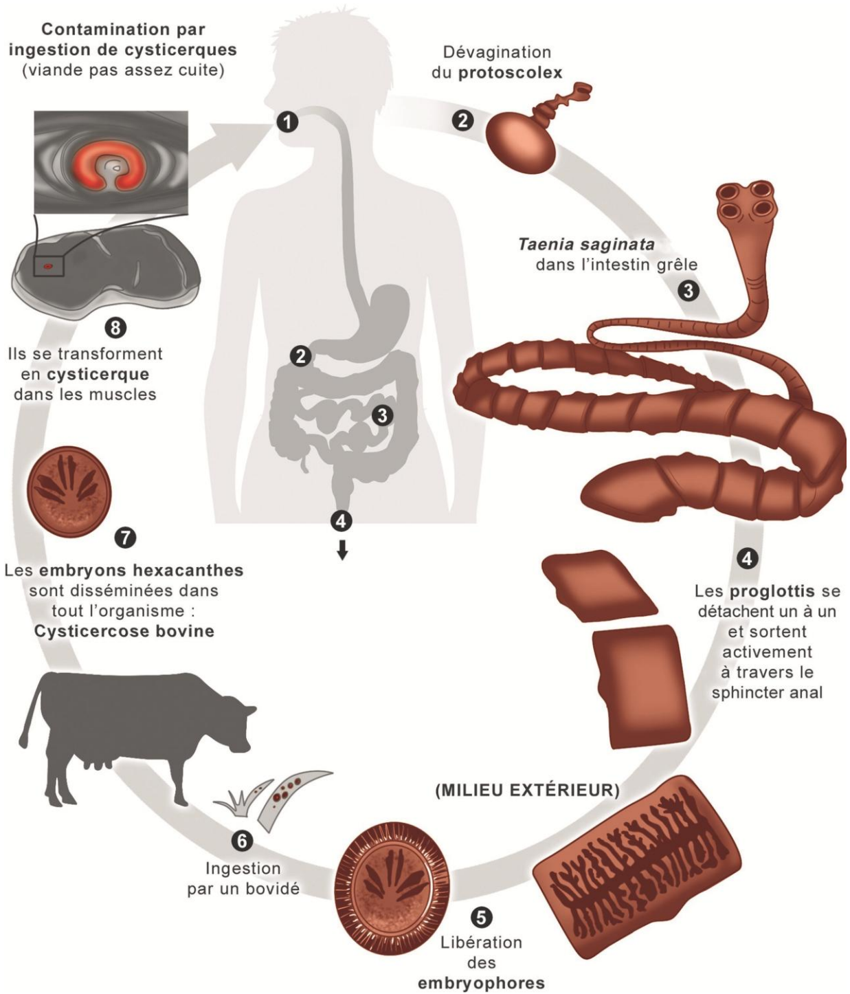
Figure 5 : Cycle évolutif de Taenia saginata ( http://campus.cerimes.fr/parasitologie/enseignement/taeniasis/site/html/1.html ).
