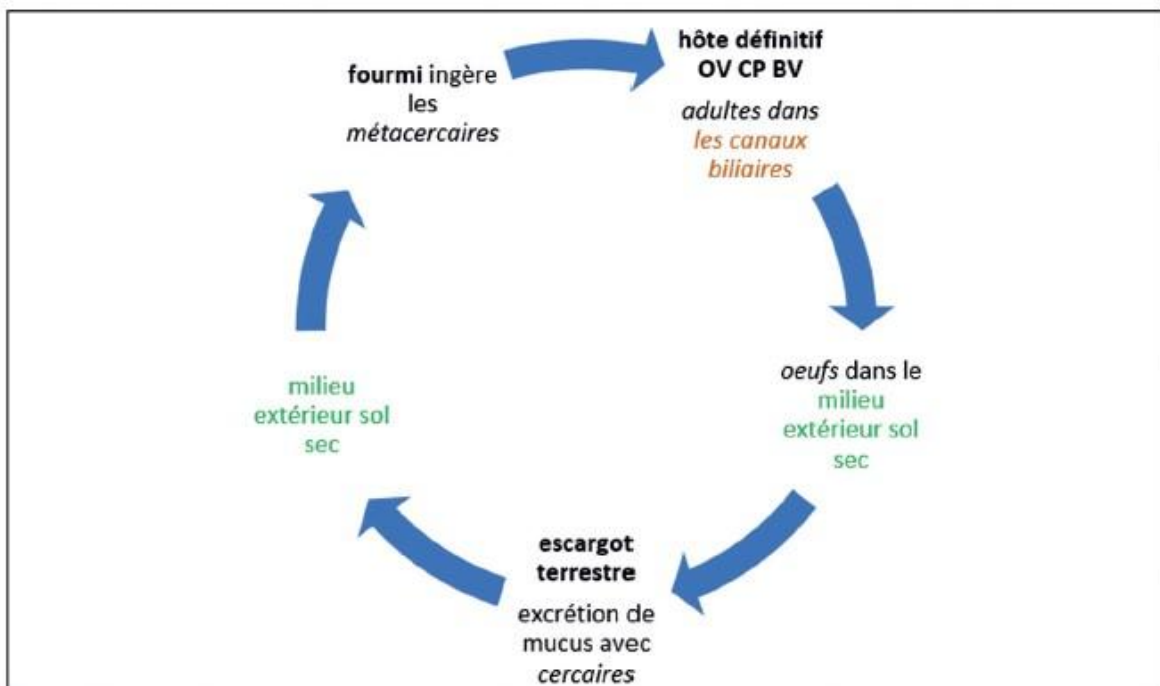
Figure 2 : Représentation schématique des étapes du cycle évolutif de la microcaeliose (petite douve) (Dubois-Frapsauce, 2019). Cycle évolutif dixène. OV : Ovins, CP : Caprins, BV : Bovins.
