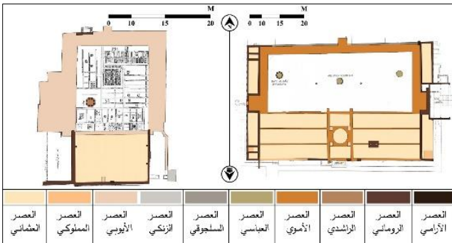
شكل (12): مقارنة المخطط التاريخي للجامع الأموي بدمشق (يمين)، وللجامع الأعلى بحماة (يسار). المصدر: الباحثة
