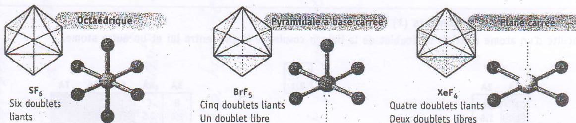
Figure 6.14 La géométrie des paires d'électrons et des molécules à atome central entouré de cinq ou six doublets électroniques.
